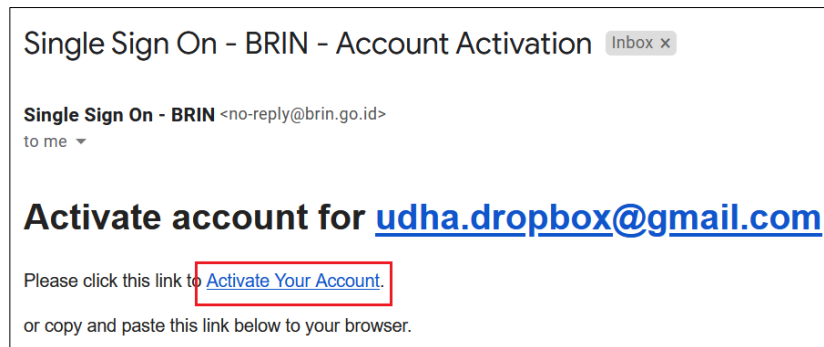
Gambar 5. Aktivasi akun
